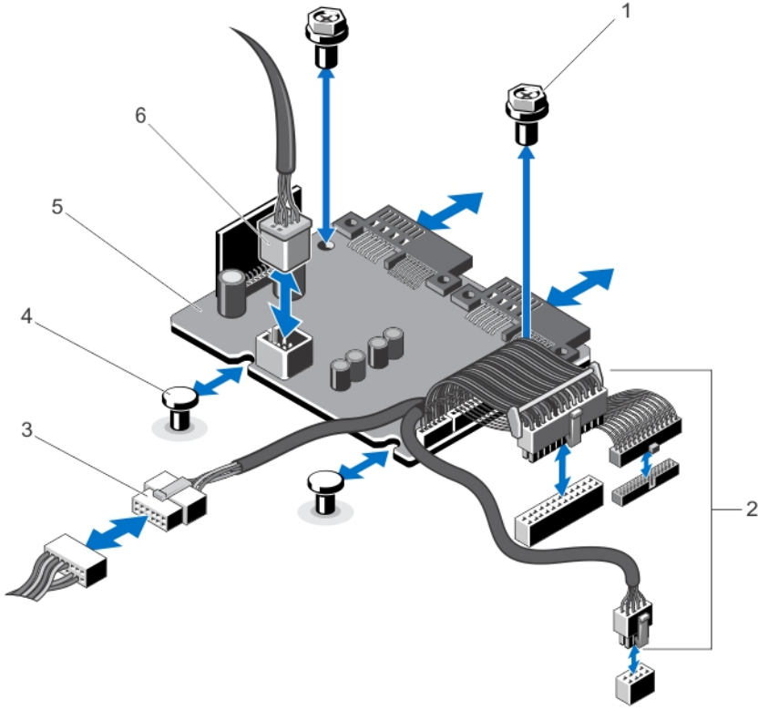
Rakam 38. Güç Dağıtım Kartını Çıkarma ve Takma
