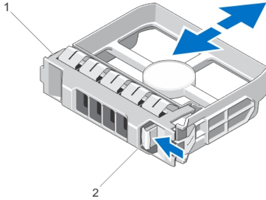
Rakam 13. 3,5 İnce Boş Sabit Sürücüyü Çıkarma ve Takma
