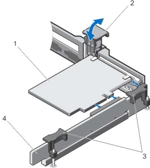
Rakam 19. Genişletme Kartı Yükselticisi 1'den Genişletme Kartını Çıkarma ve Takma
