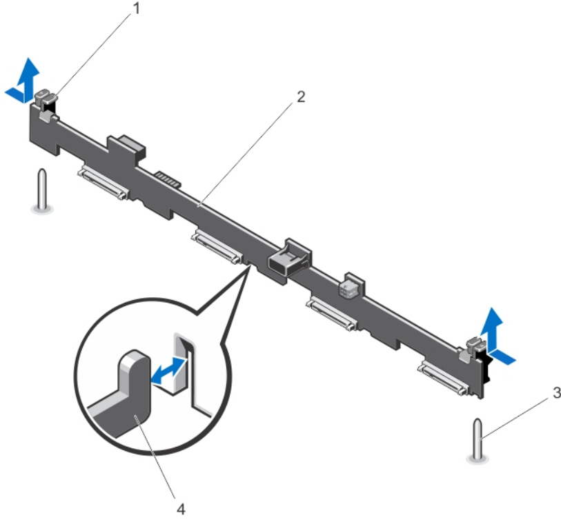
Rakam 33. Dört Sabit Sürücü Arka Paneli Çıkarma ve Takma
