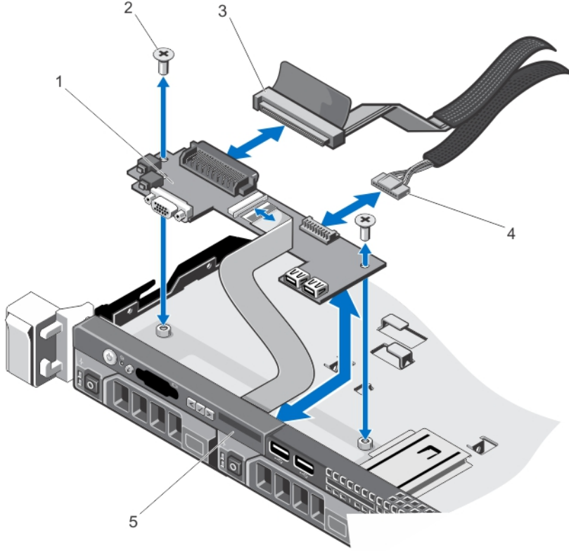
Rakam 36. Kontrol Paneli Modülünü Çıkartma ve Takma
