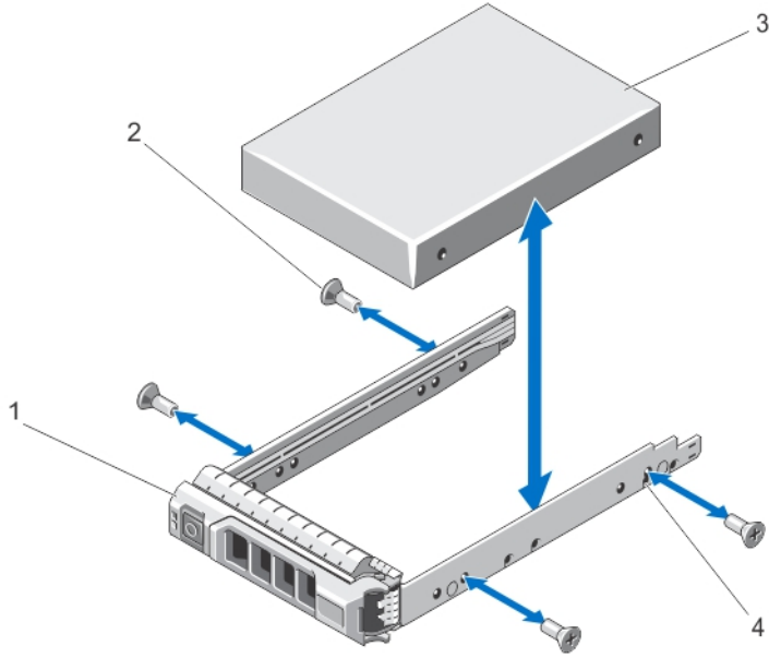
Rakam 15. Çalışırken Takılabilir Bir Sabit Sürücüyü Sabit Sürücü Taşıyıcısına Takma ve Sökme
