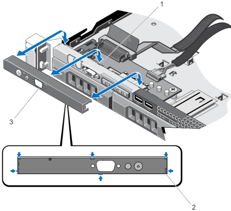
Rakam 35. Kontrol Panelini ıkarma ve Takma
