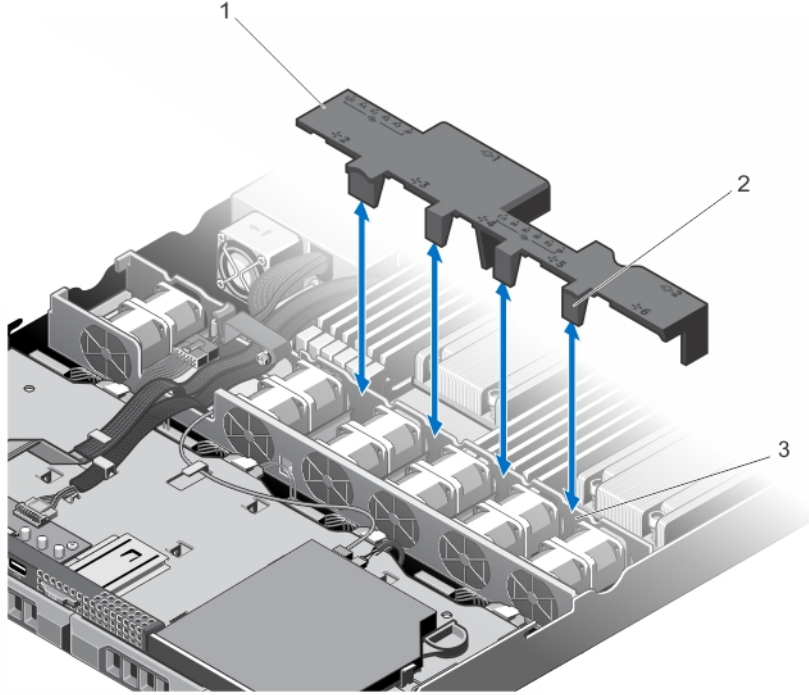
Rakam 10. Soğutma Örtüsünü Çıkarma ve Takma
