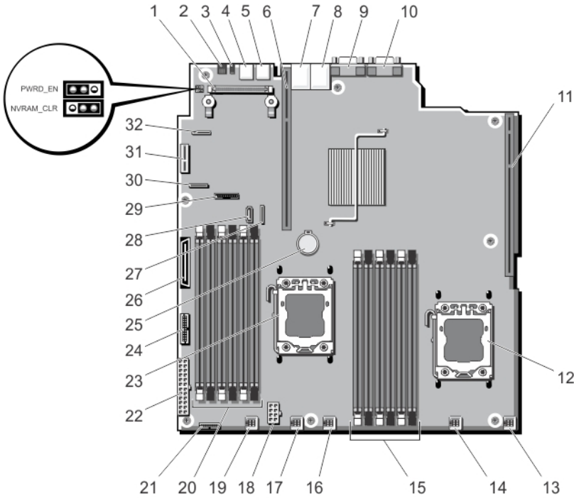
Rakam 40. Sistem Kartı Atlama Telleri ve Konektörleri
