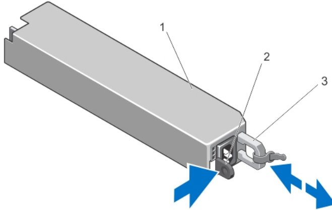
Rakam 29. Güç Kaynağını Çıkarma ve Takma
