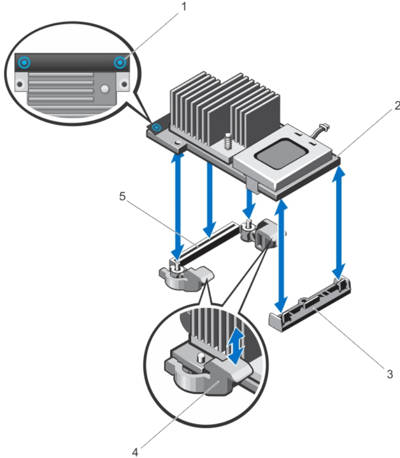
Rakam 26. Tümleşik Depolama Denetleyicisi Kartını Çıkarma ve Takma
