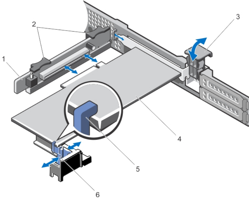
Rakam 20. Genişletme Kartı Yükselticisi 2'den Genişletme Kartını Çıkarma ve Takma
